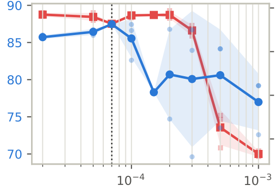
LoRA-Null
